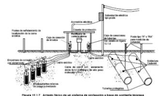
Figura 12.1.7 Arreglo típico de un sistema de producción a base de corriente impresa
